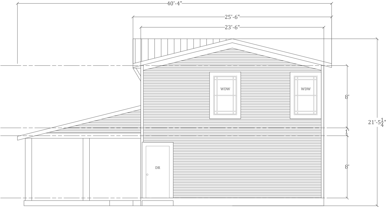
RIGHT ELEVATION
