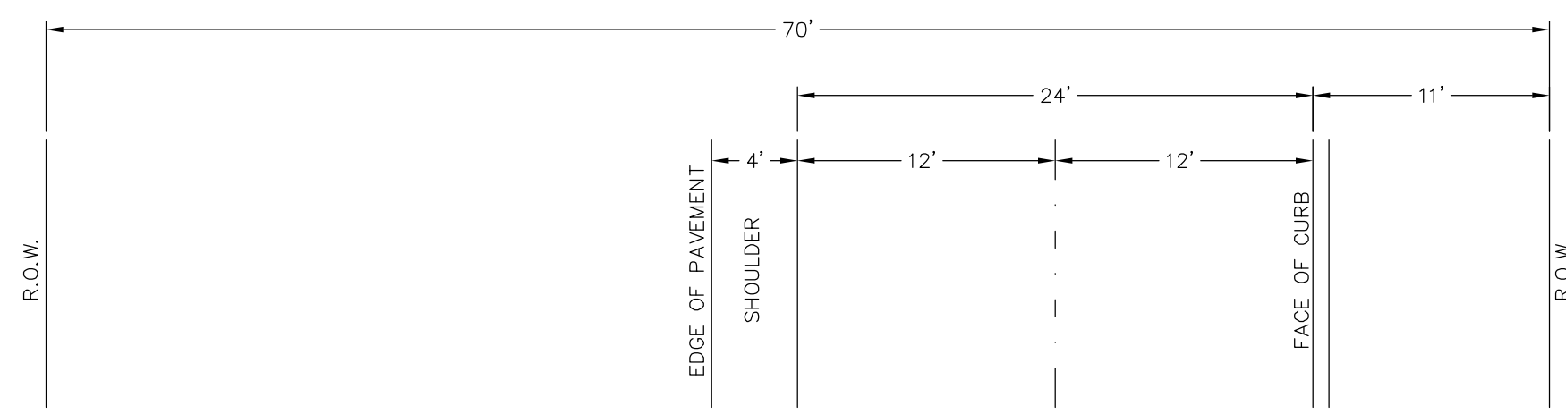
70' R.O.W. MINOR ARTERIAL N.T.S.
