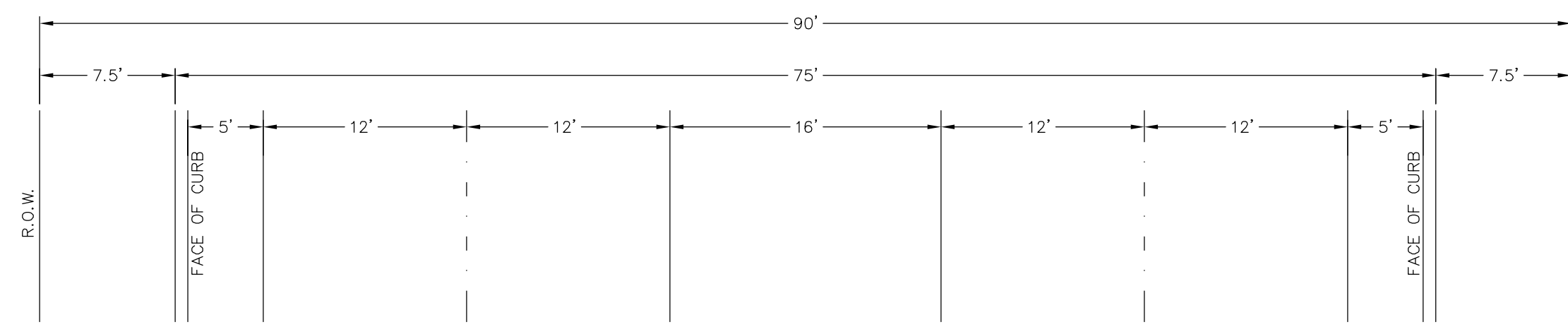
90' R.O.W. MAJOR ARTERIAL N.T.S.
